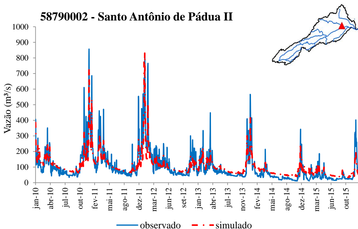
Figura 32: Hidrograma simulado e observado para o período de verificação no posto 58790002 – Santo Antônio de Pádua II e localização do posto na bacia.
