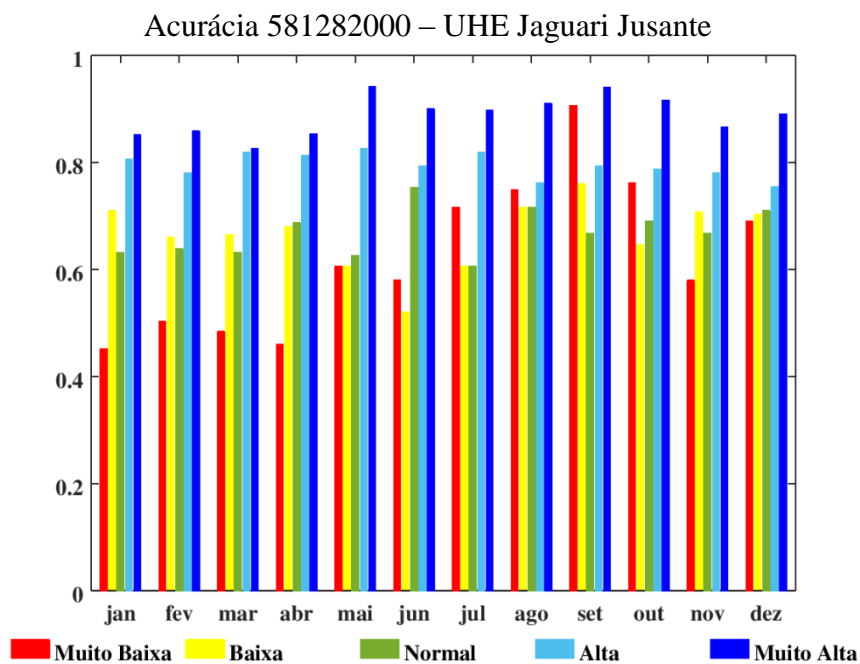
Figura D3: Acurácia mensal para o ponto 581282000 – UHE Jaguari Jusante para o período de calibração.
