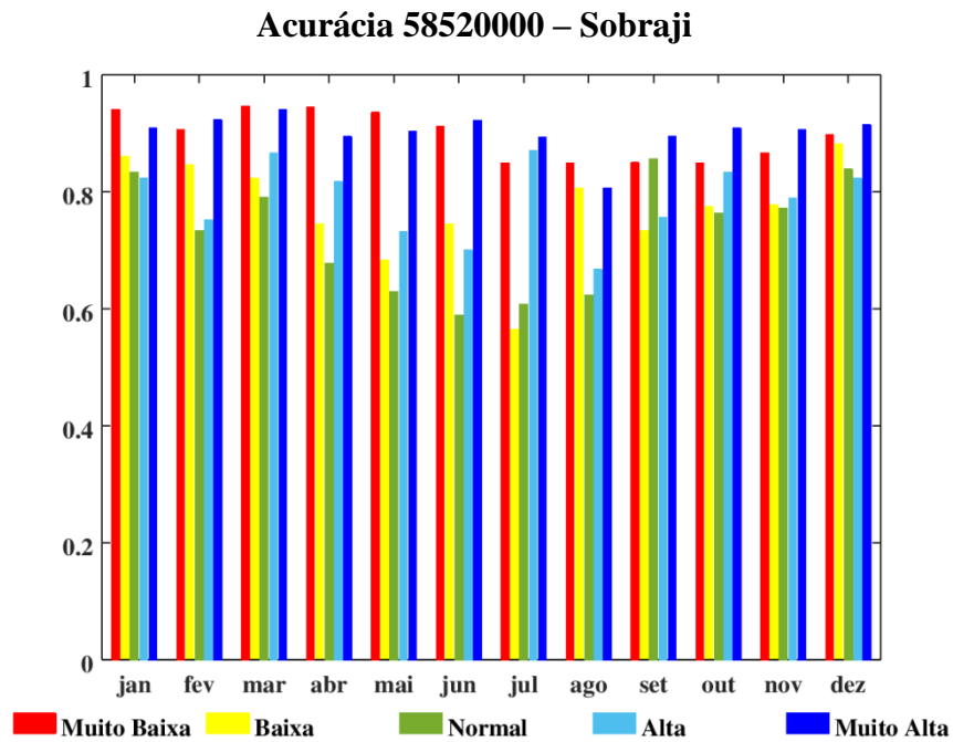
Figura 36: Acurácia mensal para o ponto 58520000 – Sobraji para o período de verificação.
