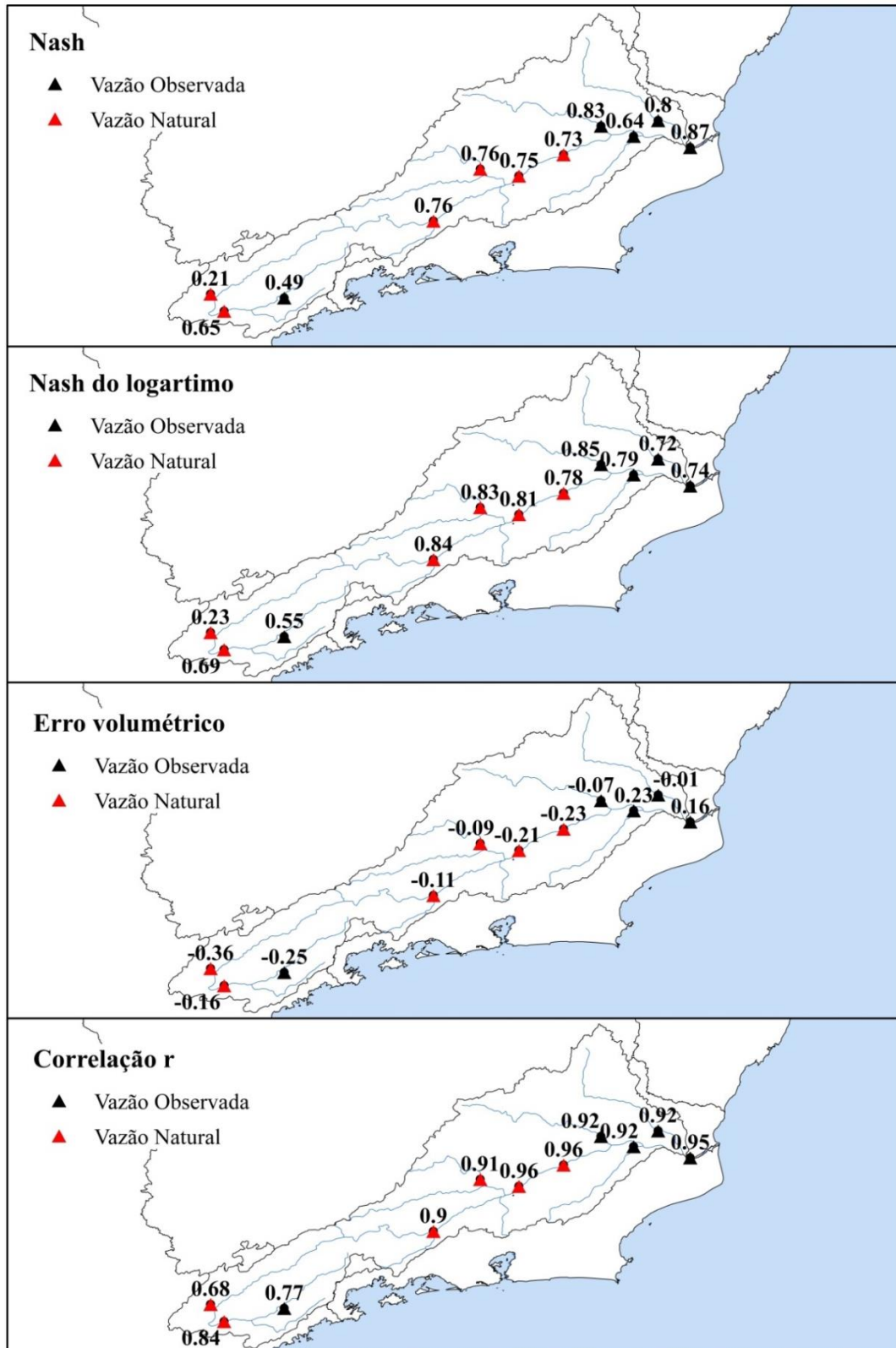
Figura 12: Disposição espacial dos parâmetros Nash ( R^2 ), Nash para o logaritmo das vazões ( Rlog ), relação entre vazões observadas e calculadas ( \Delta V ) e Correlação de Pearson ( r ) para o período de calibração do modelo.
