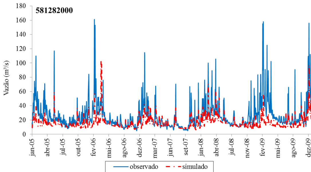
Figura C3: Hidrograma simulado e observado para o período de calibração no posto 581282000 – UHE Jaguari Jusante
