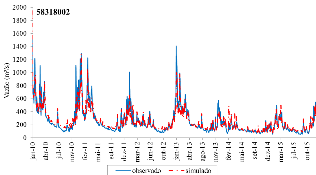
Figura C15: Hidrograma simulado e observado para o período de verificação no posto 58318002 – UEL Santa Cecília Jusante.
