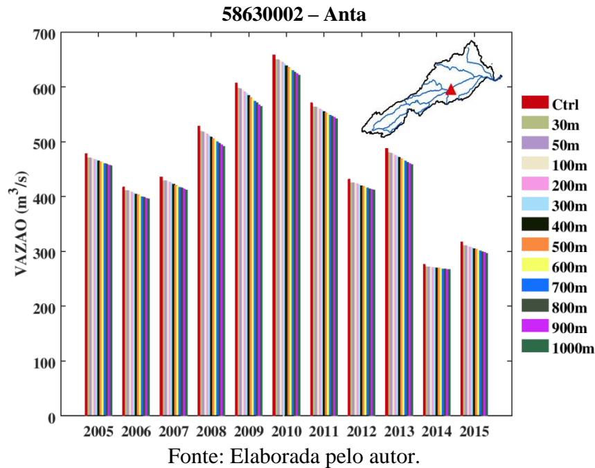
Figura 43: Vazão média anual para o cenário de controle (Ctrl na legenda) e nos cenários que consideram recomposição da vegetação ripária de 30m, 50m, 100m, 200m, 300m, 400m, 500m, 600m, 700m, 800m, 900 m e 1000m, no posto Anta.
