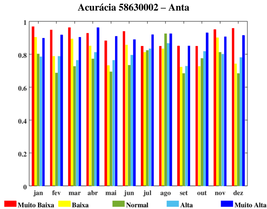
Figura 37: Acurácia mensal para o ponto 58630002 – Anta para o período de verificação.
