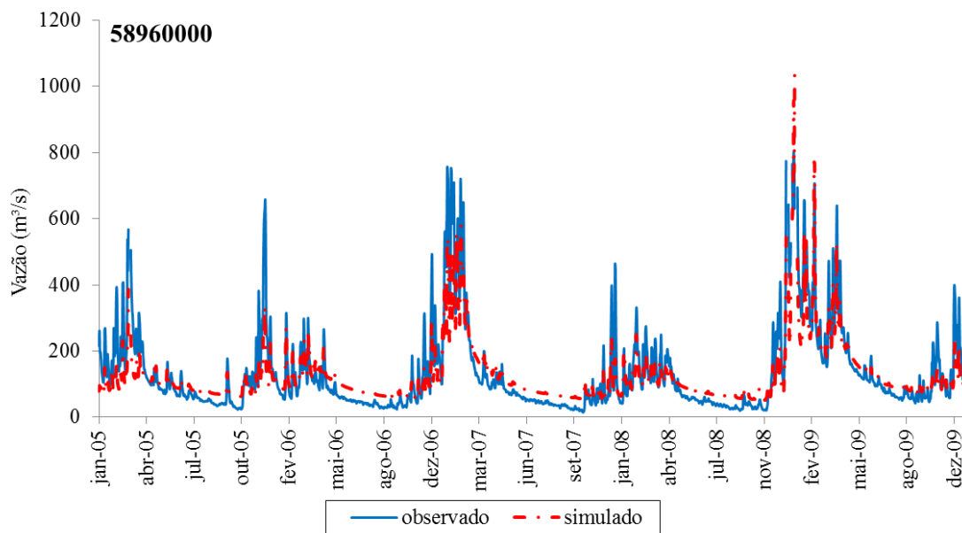
Figura C10: Hidrograma simulado e observado para o período de calibração no posto 58960000 – Cardoso Moreira
