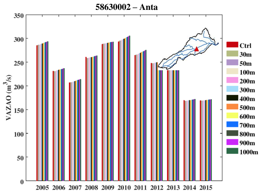
Figura 55: Vazão Q95 anual para o cenário de controle (Ctrl) e nos cenários que consideram recomposição da vegetação ripária de 30m, 50m, 100m, 200m, 300m, 400m, 500m, 600m, 700m, 800m, 900 m e 1000m no posto Anta.
