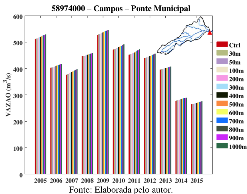
Figura 57: Vazão Q95 anual para o cenário de controle (Ctrl) e nos cenários que consideram recomposição da vegetação ripária de 30m, 50m, 100m, 200m, 300m, 400m, 500m, 600m, 700m, 800m, 900 m e 1000m no posto Campos.
