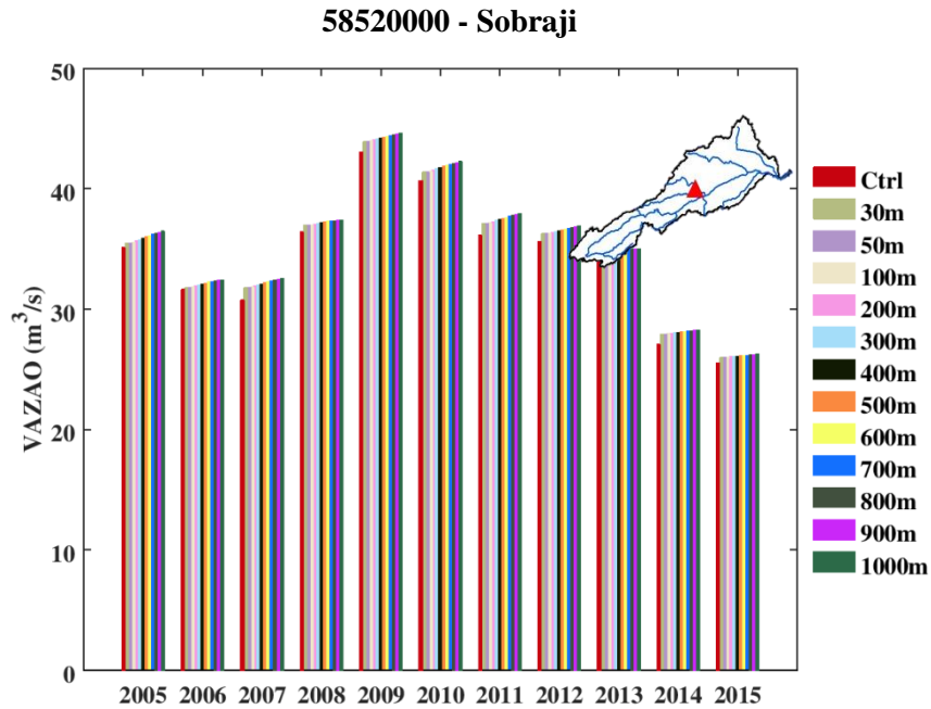
Figura 54: Vazão Q95 anual para o cenário de controle (Ctrl) e nos cenários que consideram recomposição da vegetação ripária de 30m, 50m, 100m, 200m, 300m, 400m, 500m, 600m, 700m, 800m, 900 m e 1000m no posto Sobraji.
