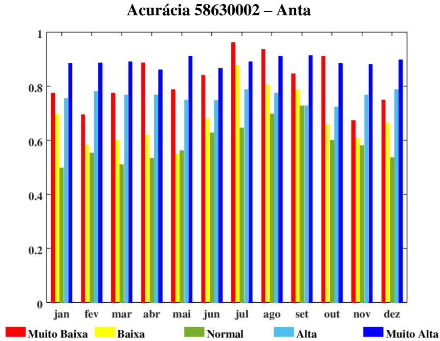
Figura 23: Acurácia mensal para o ponto 58630002 – Anta para o período de calibração.
