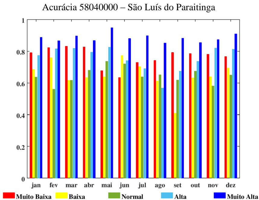
Figura D1: Acurácia mensal para o ponto 58040000 – São Luís do Paraitinga para o período de calibração
