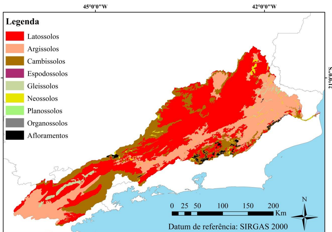
Figura 7: Mapa de solos da bacia do rio Paraíba do Sul produzido a partir de mapas de solo do Comitê de Integração da Bacia Hidrográfica do Rio Paraíba do Sul, complementado com o mapa de solos do Brasil.
