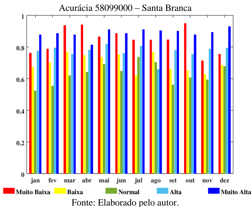
Figura D2: Acurácia mensal para o ponto 58099000 – Santa Branca para o período de calibração.
