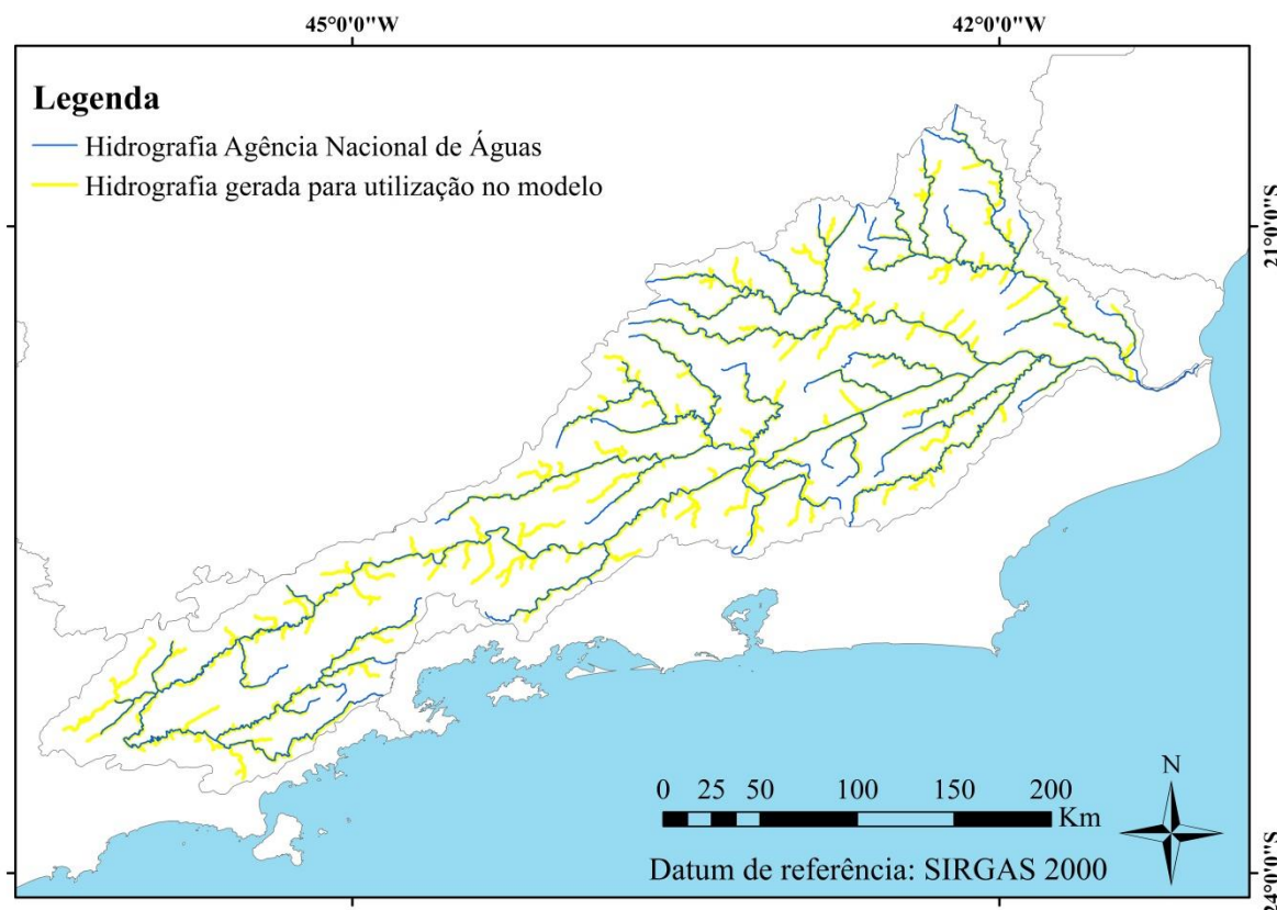
Figura 11: Comparação entre a rede de drenagem gerada para utilização no modelo, construída com base em um modelo digital de elevação (MDE) corrigido e a disponibilizada pela Agência Nacional de Águas (ANA).
