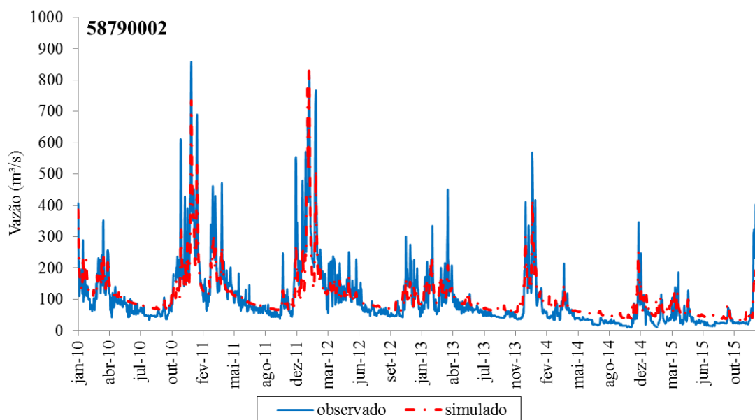
Figura C19: Hidrograma simulado e observado para o período de verificação no posto 58790002: Santo Antônio de Pádua II.
