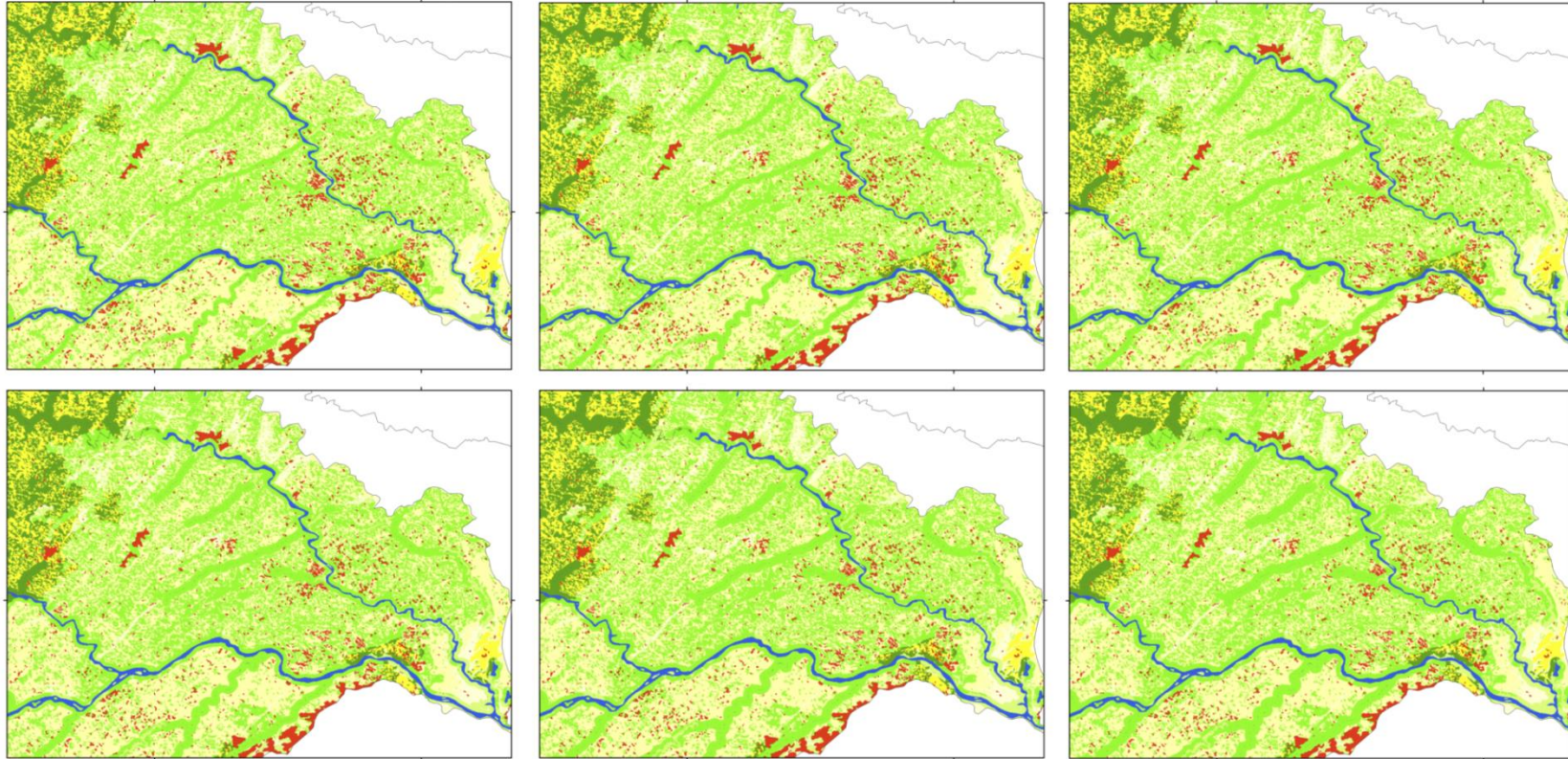
Figura A2: Unidades de Resposta Hidrológica (URH) de parte da bacia, próxima a foz do rio Paraíba do Sul, para os cenários considerando largura de vegetação marginal de 500m (a), 600m (b), 700m (c), 800m (d), 900m (e) e 1000m (f).
