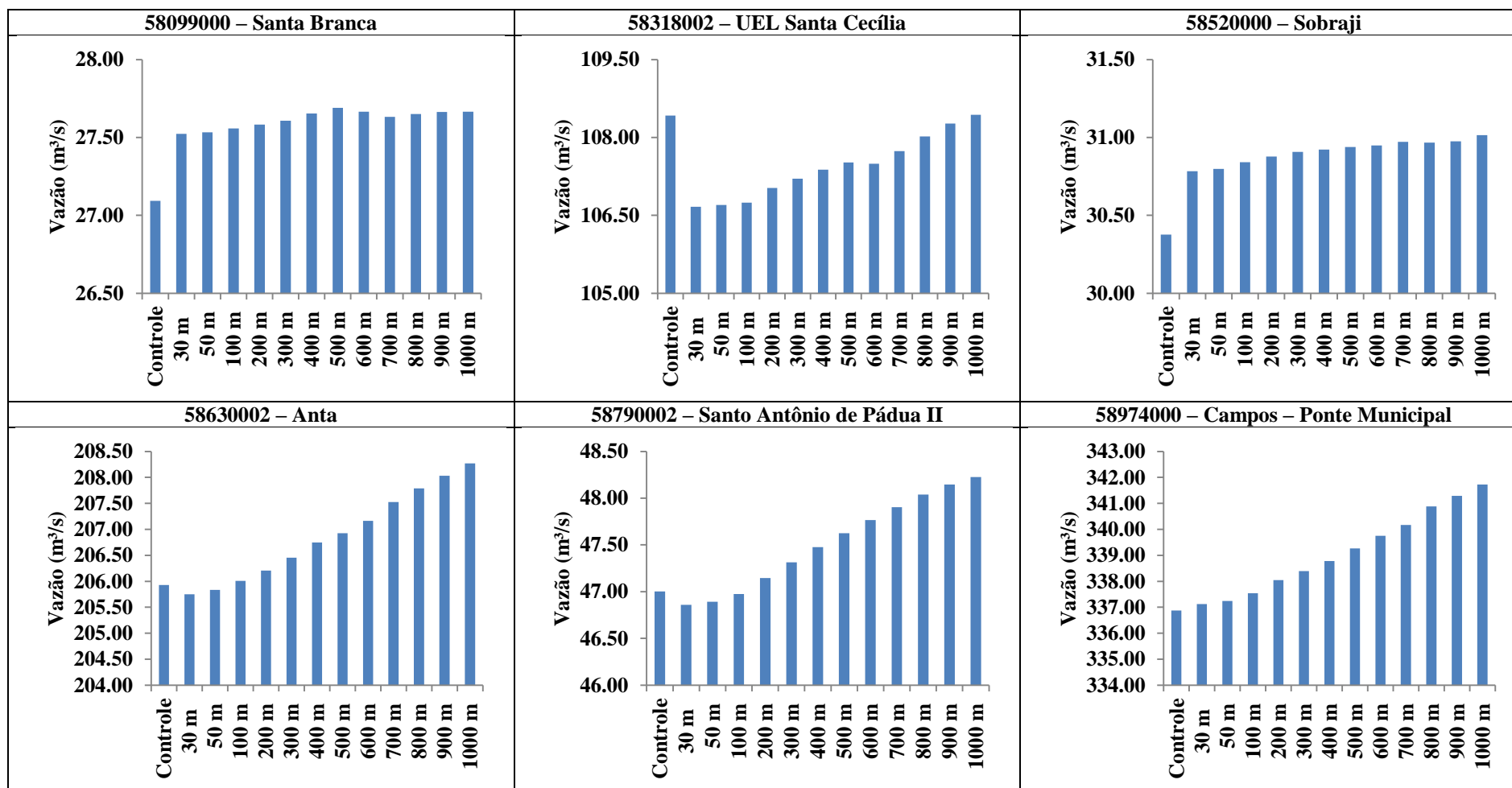
Figura 58: Vazão Q95 para todo o período de simulação, no cenário de controle (Ctrl) e nos cenários que consideram recomposição da vegetação ripária.
