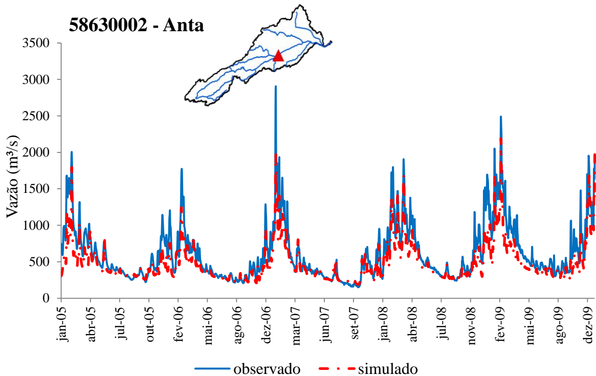
Figura 17: Hidrograma simulado e observado para o período de calibração no posto 58630002 – Anta e localização do posto na bacia.
